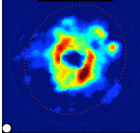
NGC4273
