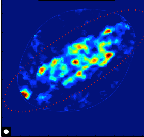
NGC6503
